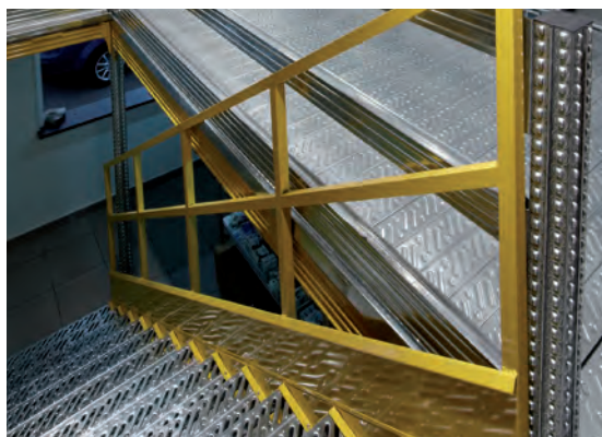
Suelo en acero pregalvanizado embutido, peldaños en acero pregalvanizado perforado.
