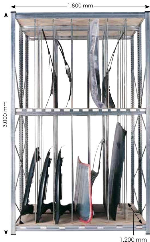
Módulo de doble fondo, total 1.200 mm.
