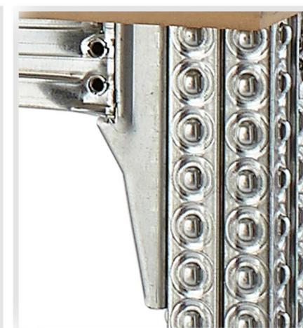
Unión a los largueros de 70 x 45 mm
